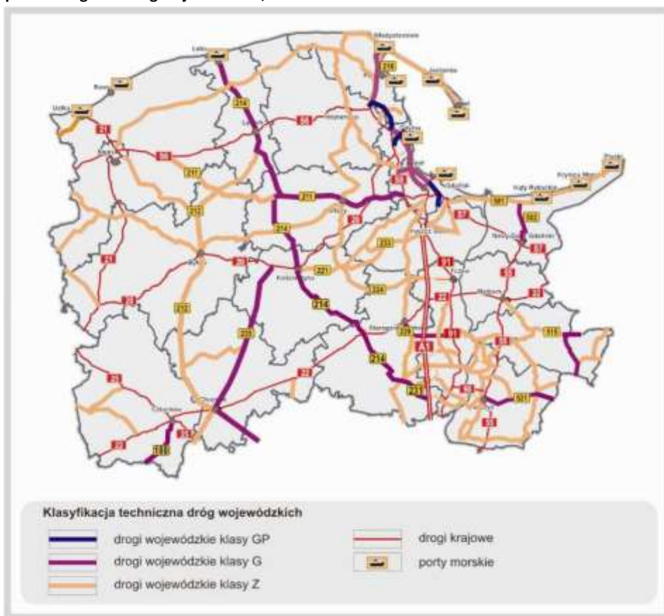
Schemat 12 Docelowe klasy dróg wg Planu zagospodarowania przestrzennego województwa pomorskiego dla dróg wojewódzkich, 2009 r.
