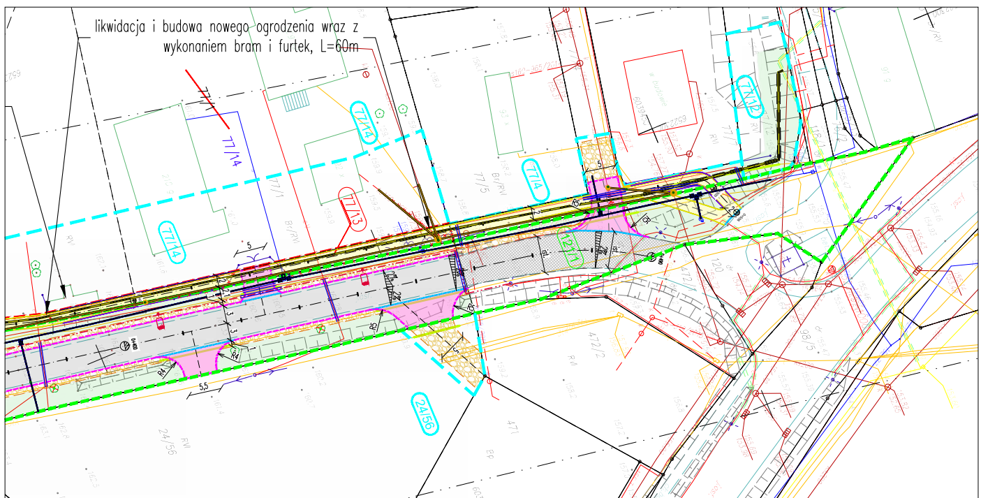
Projekt zagospodarowania terenu – ul. Kieleńska w Koleczkowie (fragment)
