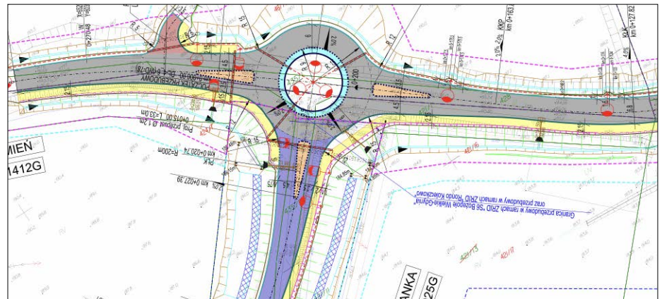
Kamień, ul. Gdańska – projekt ronda
